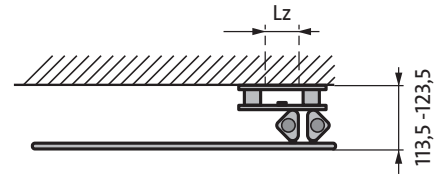
вид сверху
