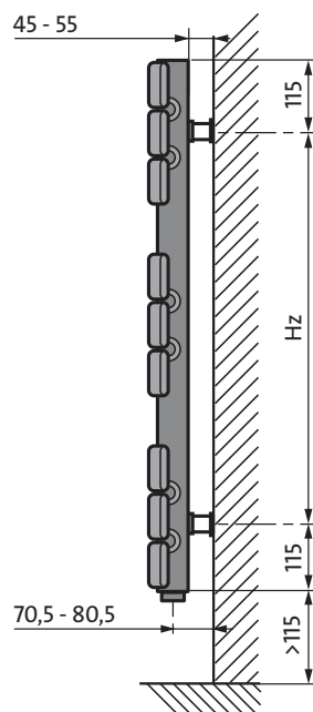
вид сбоку
