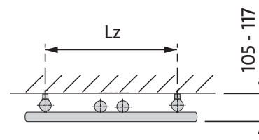
вид сверху
